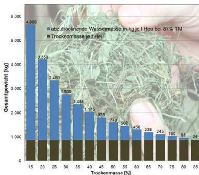
Bild 2: Die Menge des abzutrocknenden Wassers hängt stark vom Anfangs-Trockenmassegehalt ab
