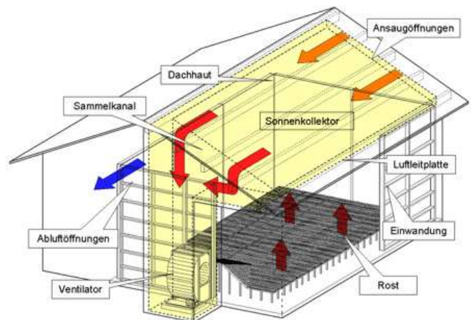
Bild 15: Heubelüftungsanlage mit ins Dach integriertem Sonnenkollektor.
