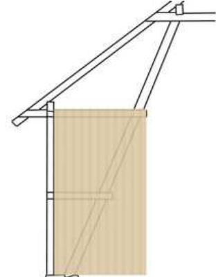
Bild 8: Nach unten fliehende Gebäudeteile verkleiden!
