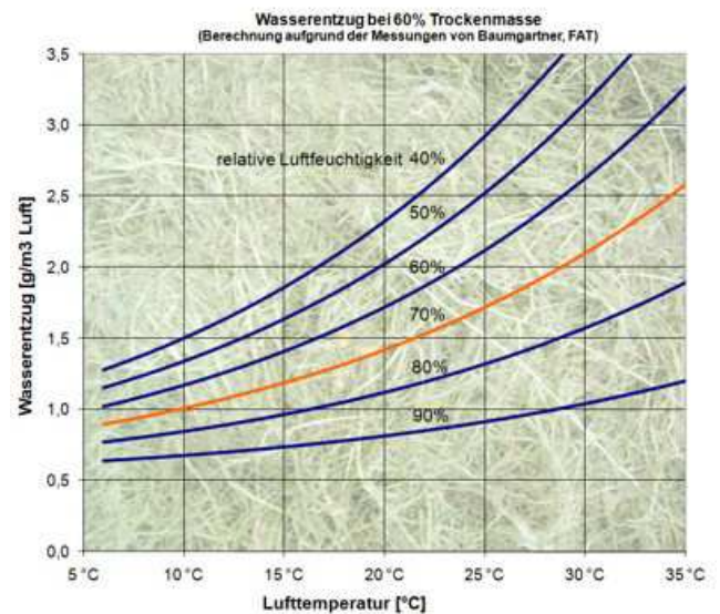
Bild 5: Maximaler Wasserentzug in g/m 3 Luft bei 60% TM
