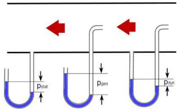
Bild 11: Druckmessung, links statischer Druck, Mitte Gesamtdruck, rechts dynamischer Druck
