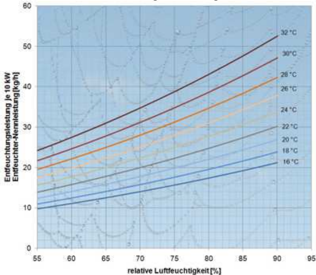
Bild 23: Die Entfeuchterleistung ist stark von der Luftfeuchtigkeit und der Temperatur abhängig! Unterhalb von 50 % rel. Luftfeuchtigkeit ist die Wirkung gering.
