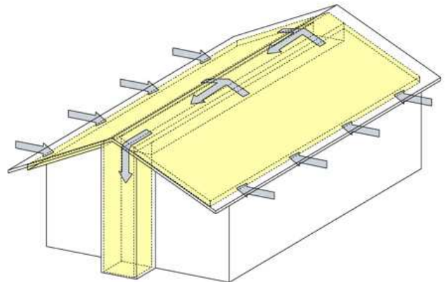
Abb. 17: Skizze einer Sonnekollektoranlage im Sparrendach mit zwei Kollektorfeldern
