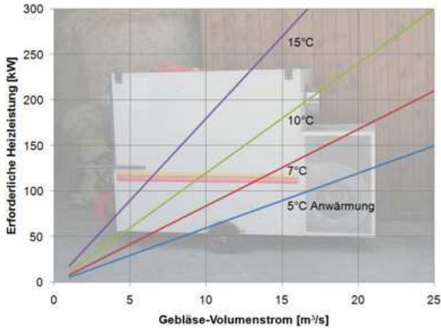
Bild 14: Erforderliche Heizleistung
