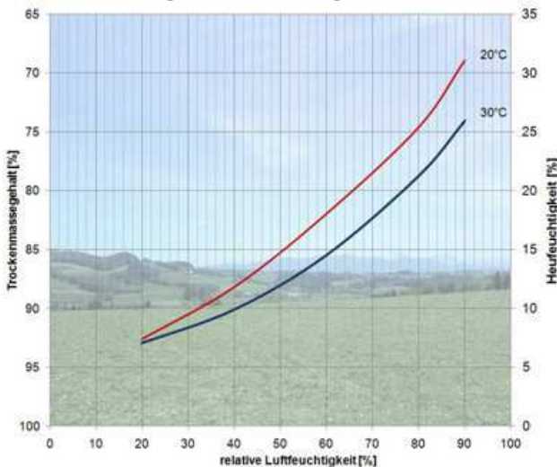
Bild 3: Feuchtigkeitsgleichgewicht von Wiesenheu (nach Segler, 1968)
