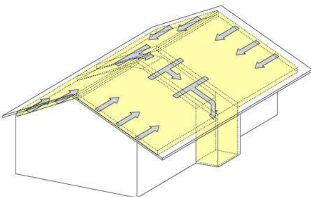
Bild 16: Sonnenkollektor im Pfettendach mit vier Kollektorfeldern auf zwei Dachflanken und einem mittigen Sammelkanal
