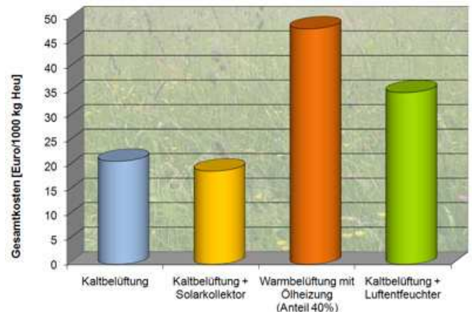
Bild 25: Gesamtkosten je 1000 kg Heu bei Trocknung von 60% auf 87% TM (Preisbasis September 2008, Stromtarif 13 Cent/kWh, ohne Kosten der Heuwerbung und ohne Gebäudekosten)
