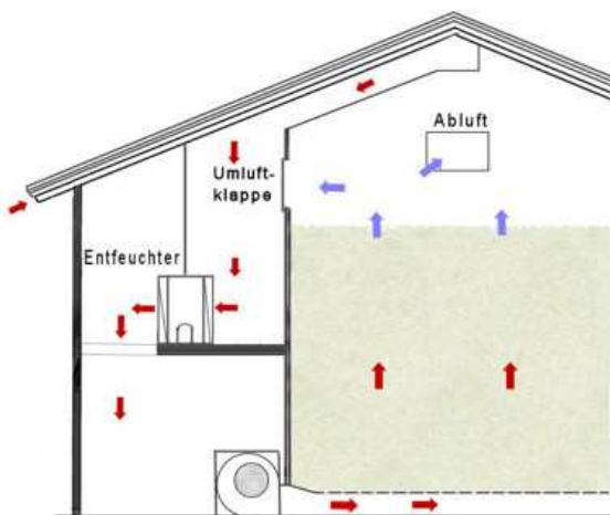
Bild 21: Anlagenschema mit Luftentfeuchter und Dachabsaugung (Variante Entfeuchtung im Hauptstrom)
