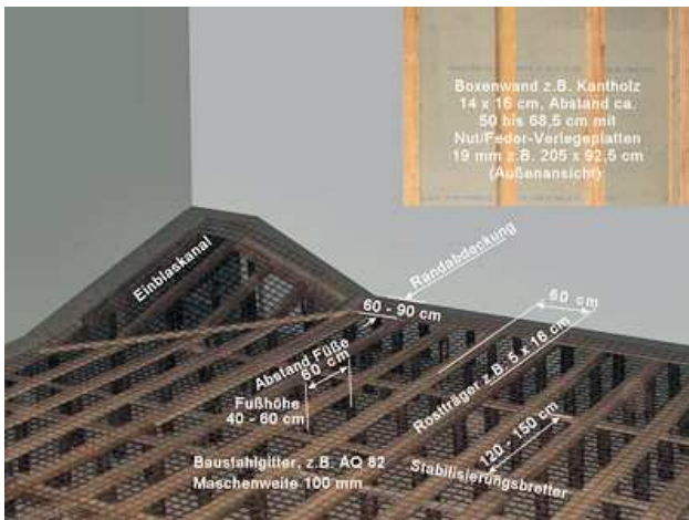
Bild 6: Beispiel für die Gestaltung des Bodenrosts. Als Rostträger werden allerdings meist Kanthölzer mit 10 x 10 cm Querschnitt verwendet
