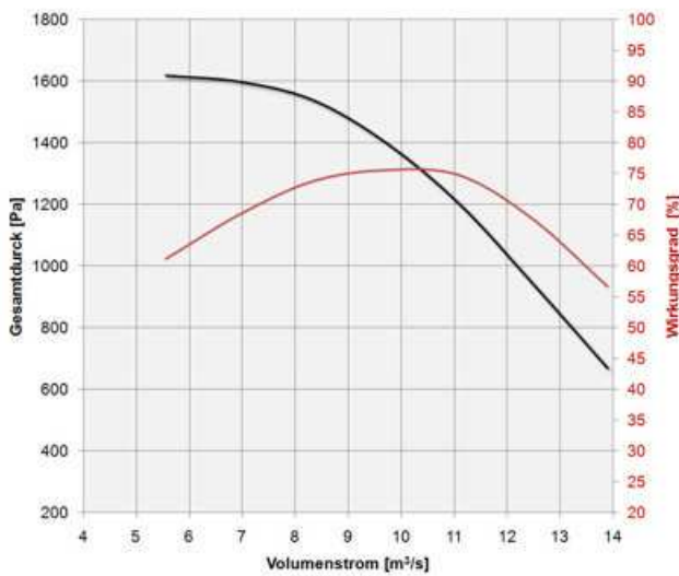
Bild 9: Kennlinien eines Ventilators für 18 kW Motornennleistung
