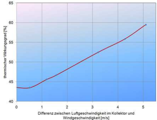
Bild 20: Die Differenz zwischen der Luftgeschwindigkeit im Kollektorkanal und der Windgeschwindigkeit sollte im Hinblick auf einen hohen thermischen Wirkungsgrad möglichst groß sein (Versuchsergebnisse der ART)
