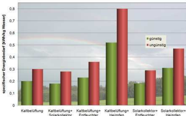
Bild 24: Spezifischer Energiebedarf verschiedener Verfahren
