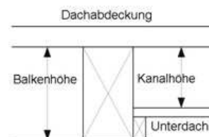
Bild 18: Die Kollektorkanäle bestehen in der Regel aus den Balken (Pfetten oder Sparren), der Dachabdeckung und der Luftleitplatte (Unterdach). Die optimale Kanalhöhe wird ausgehend von der maximalen Balkenhöhe berechnet.
